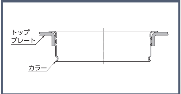
トッププレート、カラー 断面イメージ図
