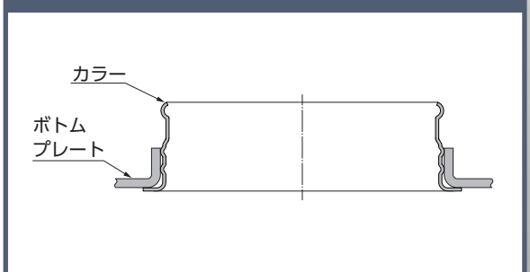
ボトムプレート、カラー 断面イメージ図
