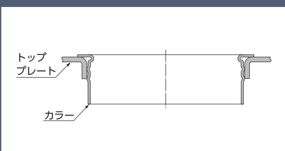
スナップタイプ プレート、カラー 断面イメージ図
